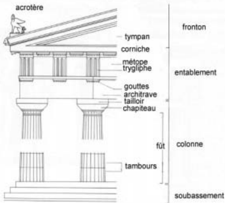
Ordre dorique avec son entablement
