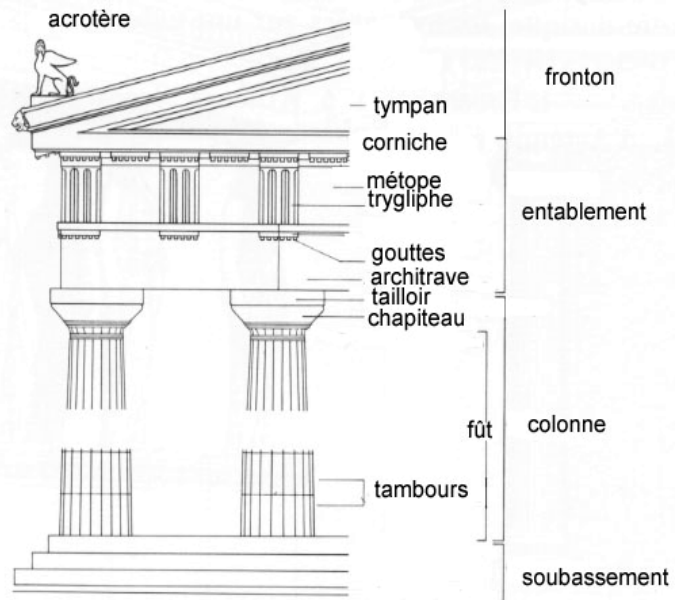
Ordre dorique avec son entablement
